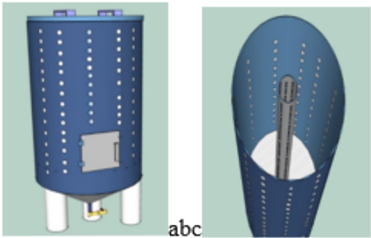
Hình 1: Bản vẽ thiết kế của thùng ủ
